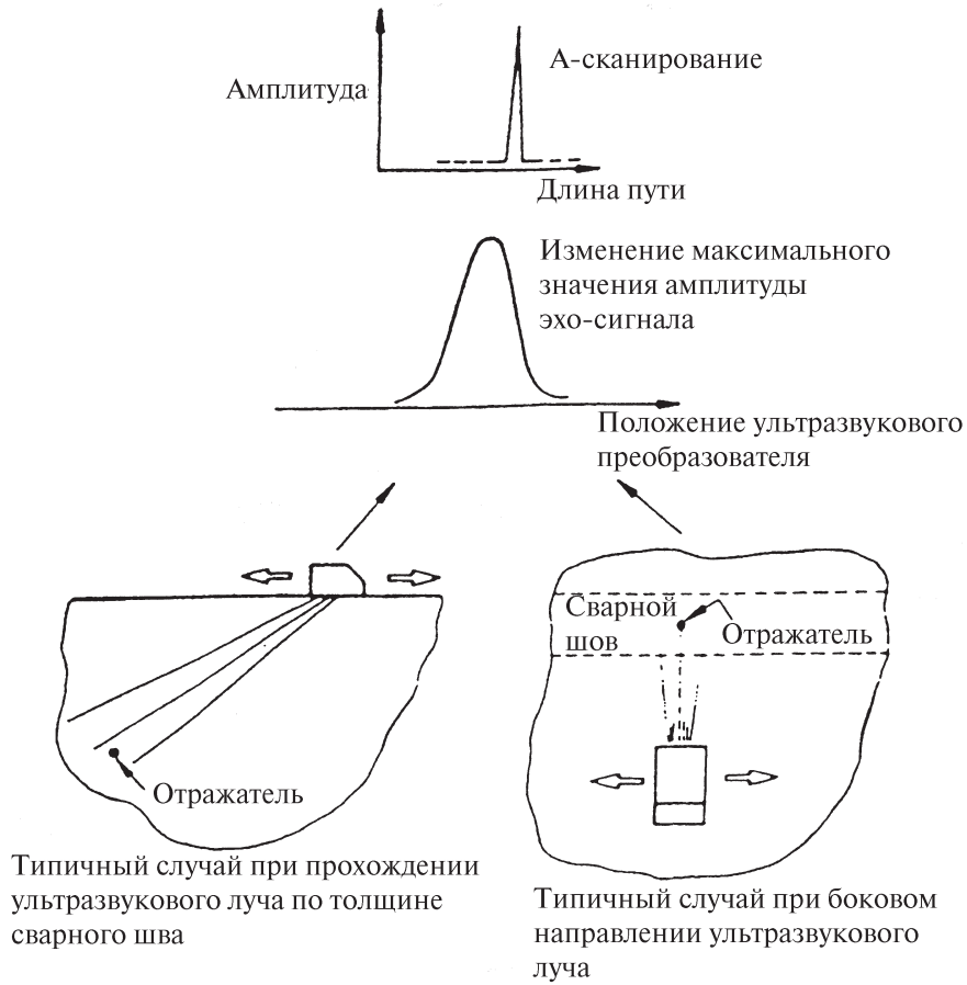
Рис. С.1. Форма 1 ультразвукового эхо-сигнала
